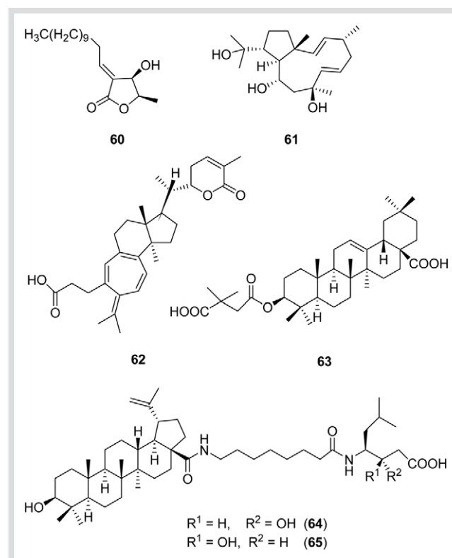
Fig. 8 Terpenes.
